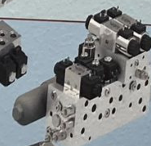
Circuito Hidráulico Integrado.
