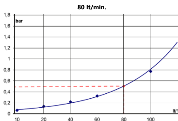
Esempio: PERDITE DI CARICO Example: PRESSURE DROP
