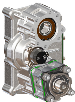
Tdf serie HIGH-POWER para transmisiones ZF TRAXON.
