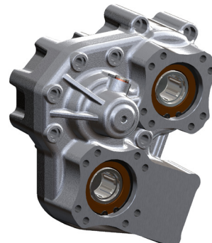
Tdf serie POWER-PLUS para transmisiones SCANIA.
