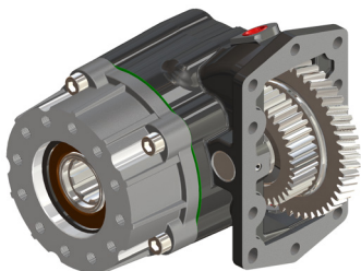
Tdf embrague eléctrico-hidráulico para transmisiones ALLISON.
