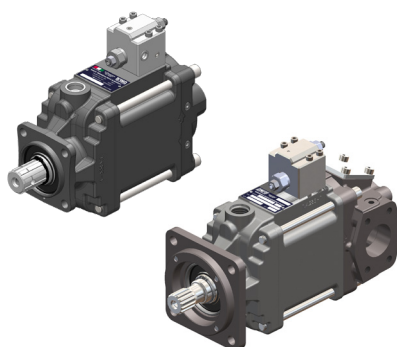
Bombas de pistones caudal variable "PPV".
