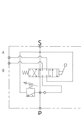
1 leva/lever
