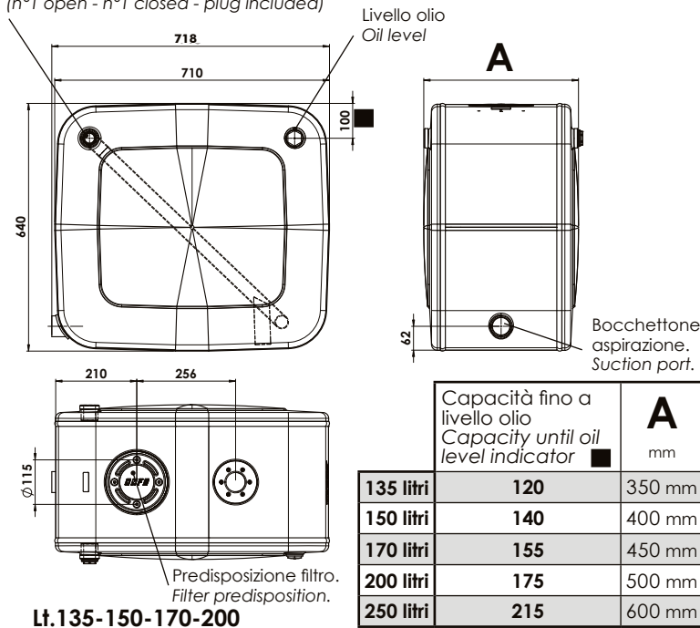
Montaggio laterale Side mounting
