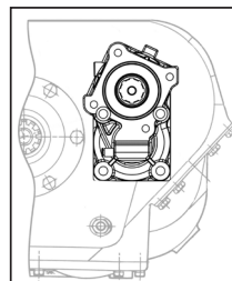
PTO MONTAGE Vertical-Sortie haute
