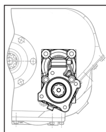
PTO MONTAGGIO Verticale-Uscita bassa
