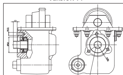
Eje macho 6x21x25 (ISO14) Salida delantera
