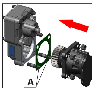
2 - Dopo aver montato la PTO al cambio, avvitare i prigionieri (pos. A) nella PTO ed inserire il gruppo appena montato (fig. 1), interponendo la guarnizione a corredo. Fissare la pompa con coppia di serraggio indicata in TABELLA 3 Cap.3.
