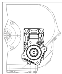
PTO MONTAGE Vertical-Sortie basse
