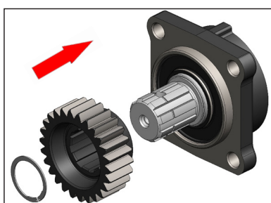
1 - Montare l'ingranaggio fornito a corredo sull'albero pompa e bloccarlo con il seeger.
