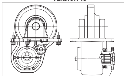
Eje macho 8x32x36 (ISO14) Salida trasera. Esta versión requiere siempre el uso de la brida (114...)
