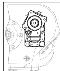
PTO MONTAGE vertikal – Ausgang oben
