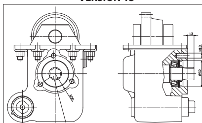
Eje macho 6x21x25 (ISO14) Salida trasera
