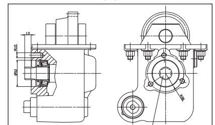
Arbre mâle 6x21x25 (ISO14) Sortie avant
