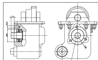
Einsteckwelle 6x21x25 (ISO14) Ausgang vorne
