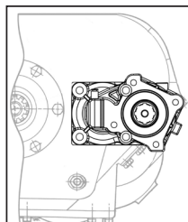
PTO MONTAGE Horizontal
