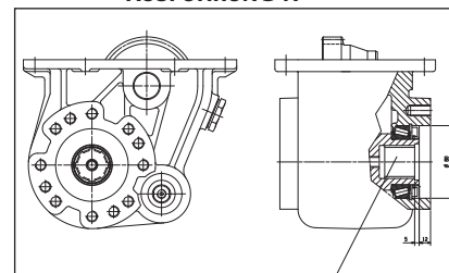
Nabe 8x32x36 (ISO14) Ausgang hinten
