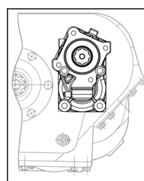
PTO MONTAGGIO Verticale-Uscita alta
