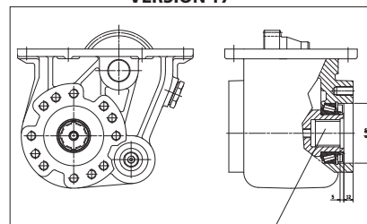
Buje hembra 8x32x36 (ISO14) Salida trasera
